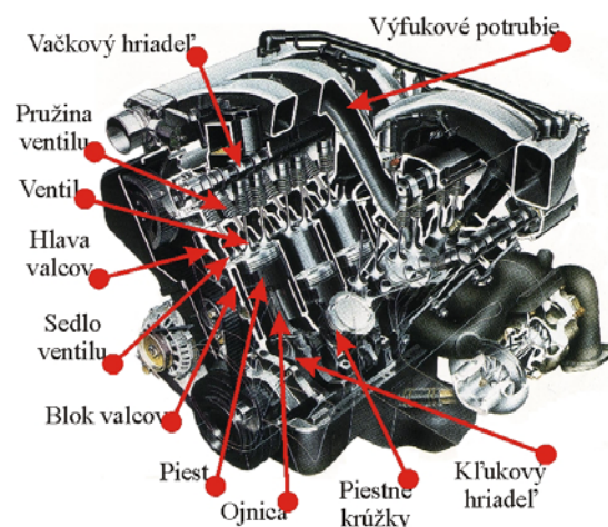
Obr. 1: Motor s popisom základných častí.
